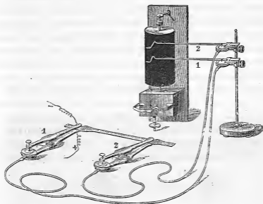
Fig. 7. — Disposition d'un faisceau musculaire entre deux pinces myographiques. La pince n° 1 porte les excitateurs électriques du muscle. — Une onde est représentée au moment où elle vient de traverser chacune des pinces.
